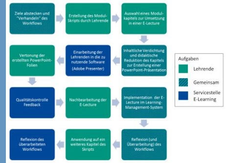
Entwicklungs-Workflow
